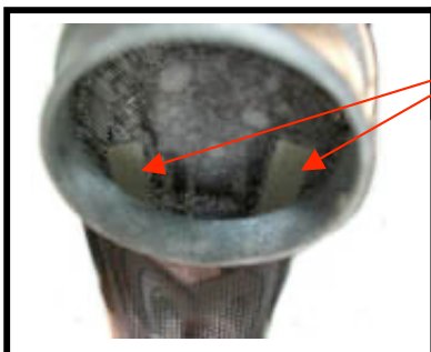
Fig : N°3 Toiles insérées Atténuent le bruit
